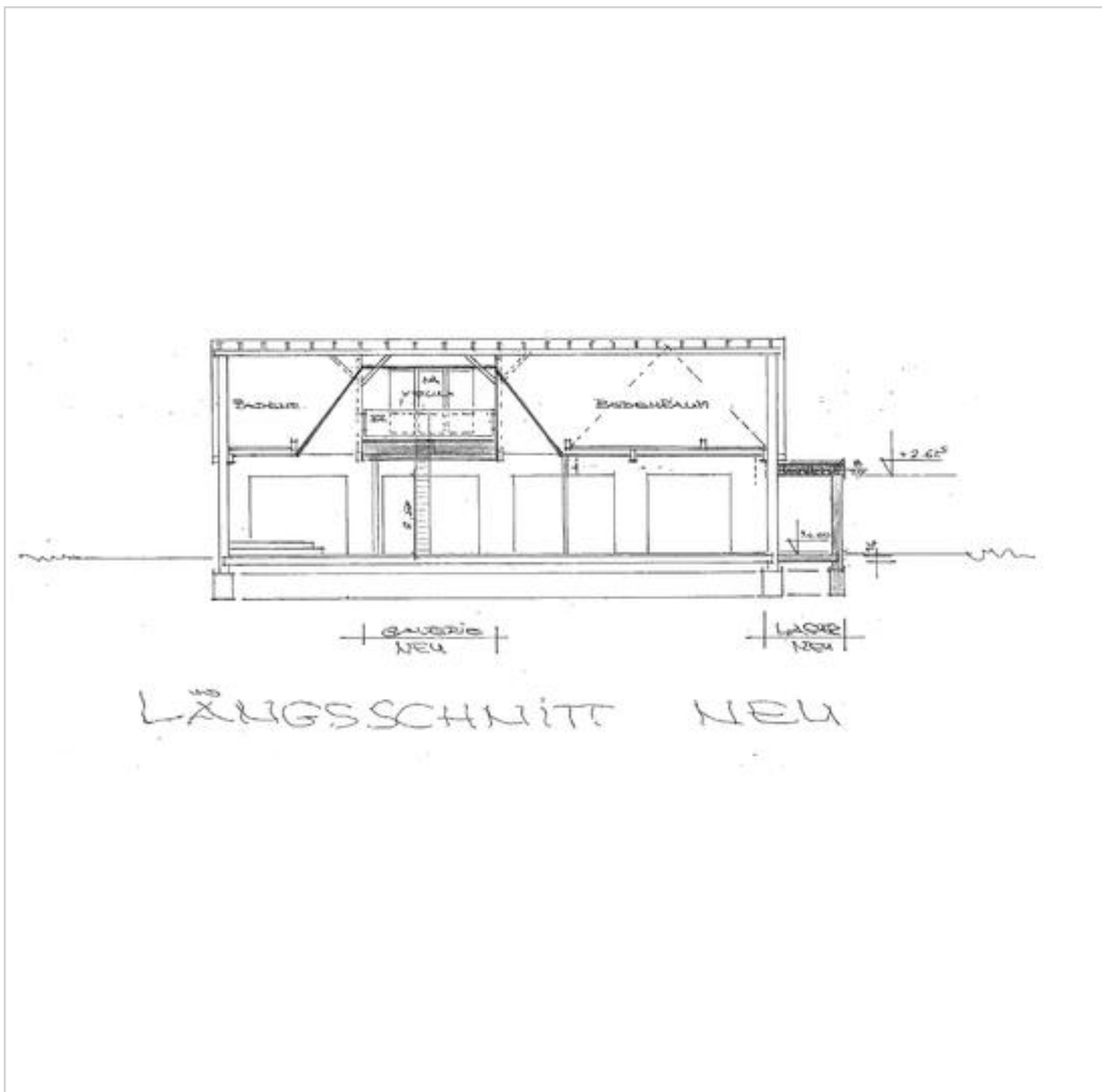
Zeichnung Längsschnitt
